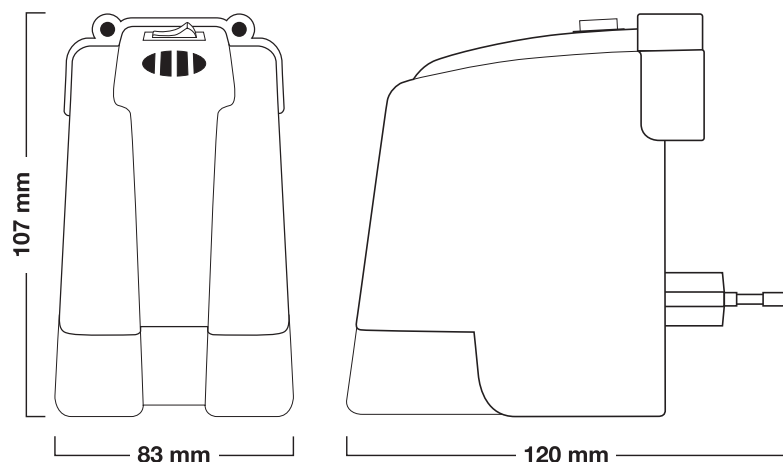
AMB 110 / 111 (Antirrobo - Antithief)
