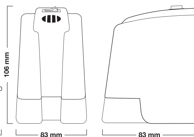
AMB 120 / 121 (Antirrobo - Antithief)
